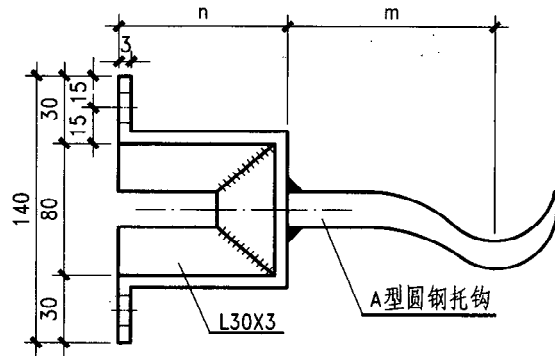
C型托钩
