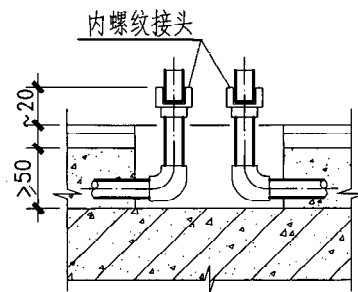
A-A 剖面
