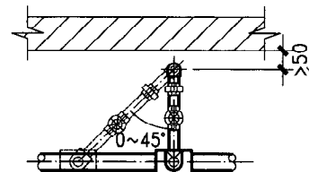
地沟内安装 B 式
