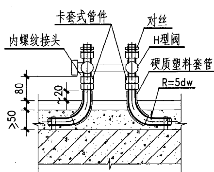
A-A 剖面
