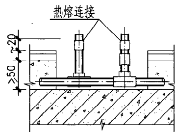
A-A 剖面
