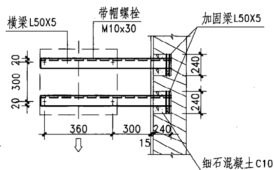
墙上安装
