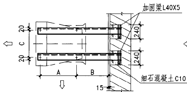
墙上安装
