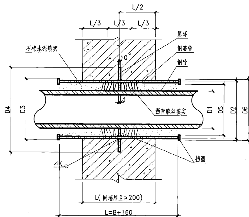
B 型
