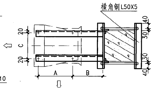
柱上安装(包箍式)
