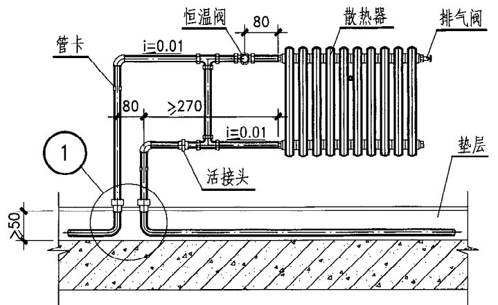
立面图
