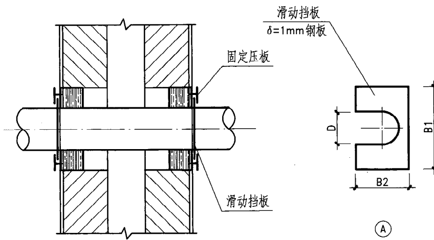
平面
