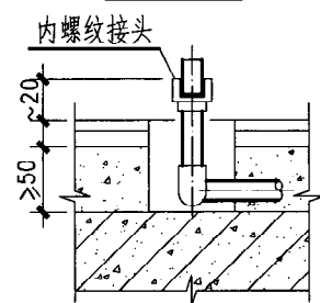
B-B剖面
