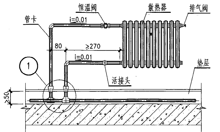
立面图
