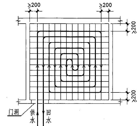
回折型布置
