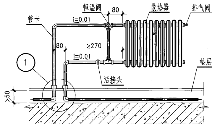
立面图
