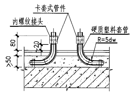
A-A 剖面
