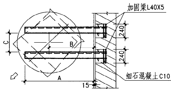
墙上安装
