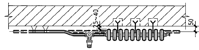
平面图
