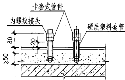
A-A 剖面
