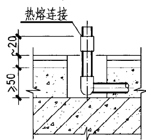
B-B剖面
