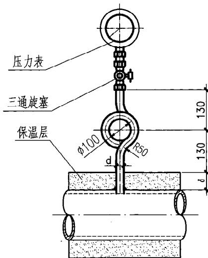
压力表在水平管上安装(上部)
