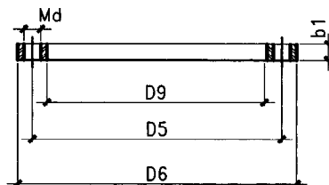
⑨ 翼盘
