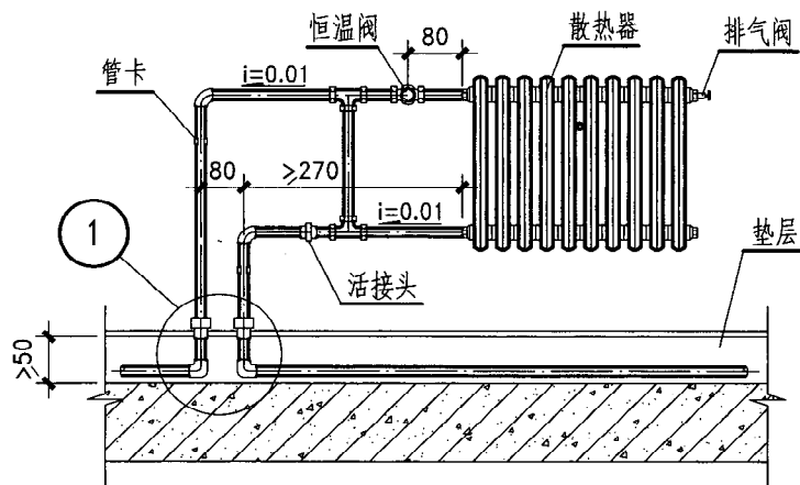
立面图
