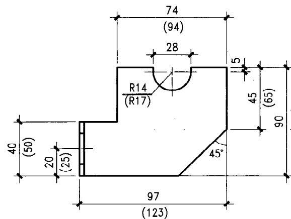
G型托架
