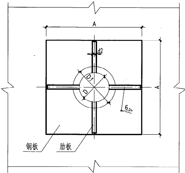
A 向视图
