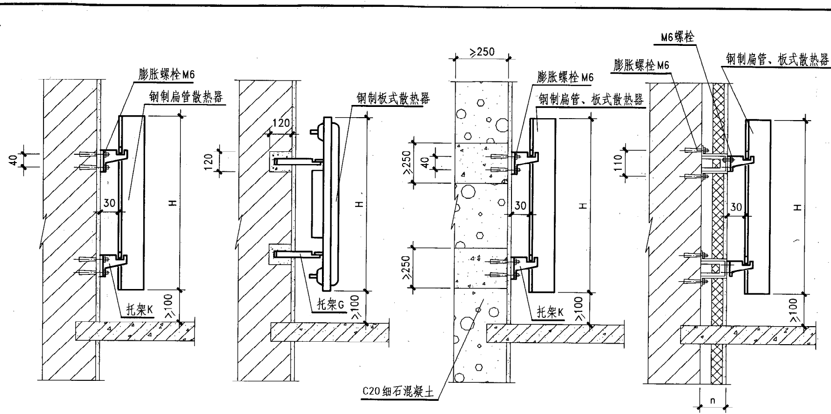
砖墙上挂装 (一)
