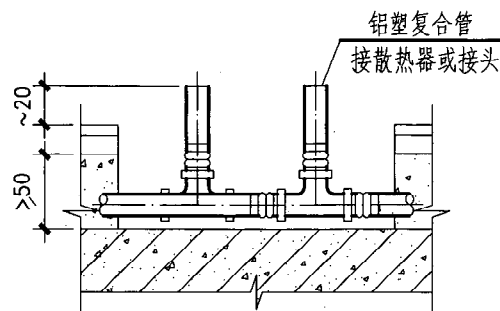
A-A 剖面
