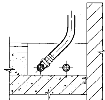
B-B 剖面
