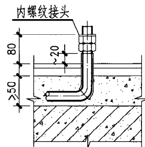
A-A 剖面
