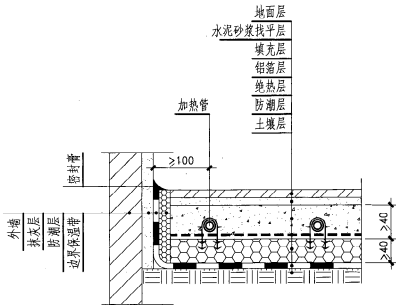
地面层辐射采暖地板构成（卡钉固定）
