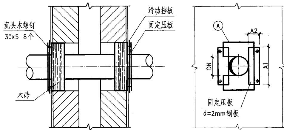
立面
