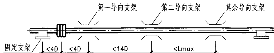
轴向式波纹伸缩节固定支架和导向管架的分布示图
