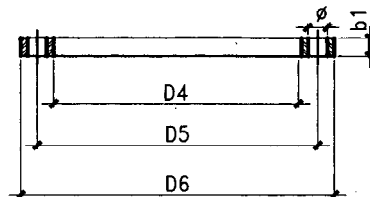
⑦ 法兰盘
