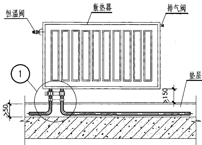
立面图
