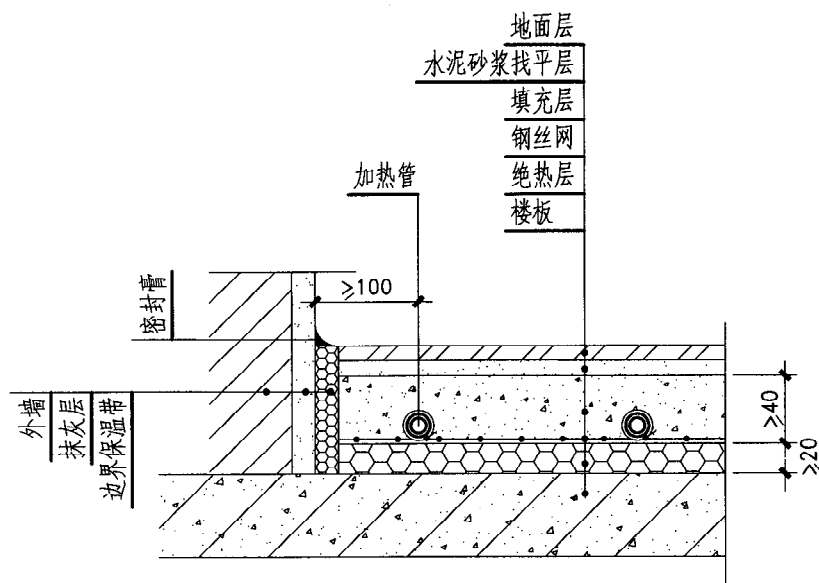
楼层辐射采暖地板构成（扎带绑扎）
