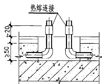
A-A 剖面
