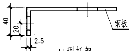
H型托架
