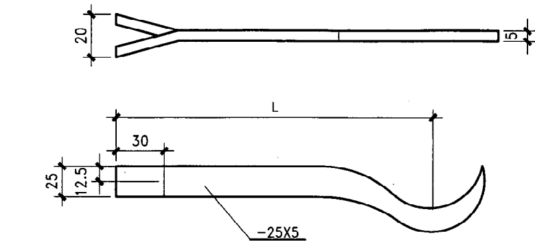
A型扁钢托钩
