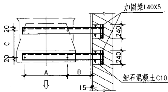
墙上安装
